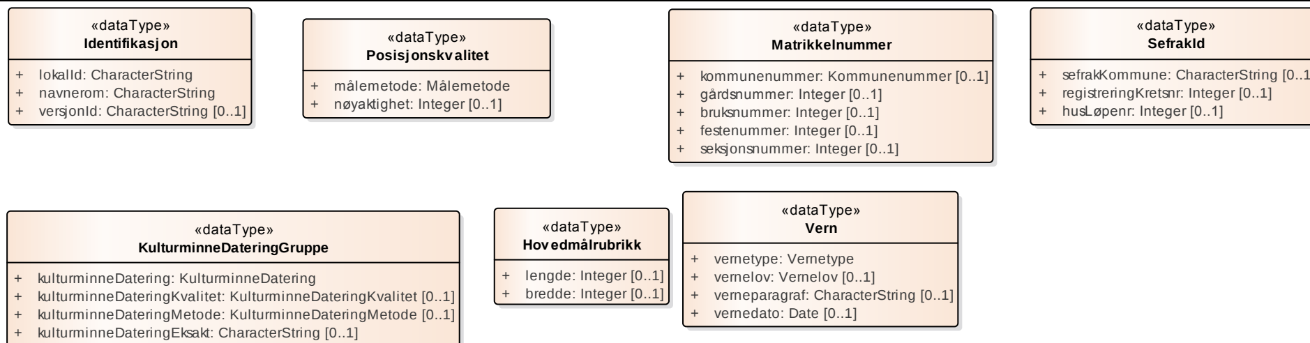
Figur 3 Datatyper
